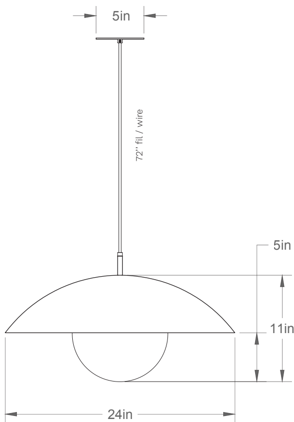
Avant/Front
