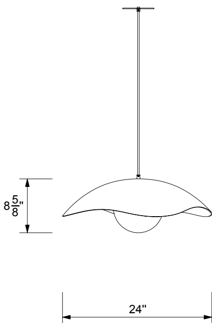
Avant / Front
