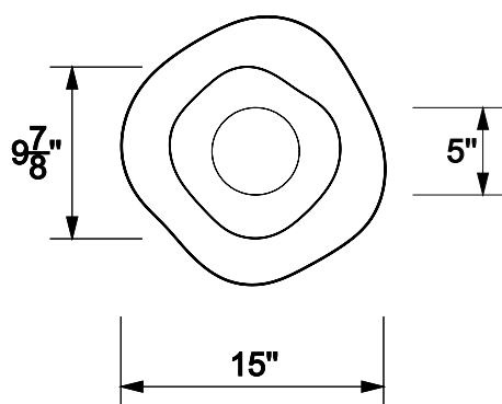
Dessous / Bottom
