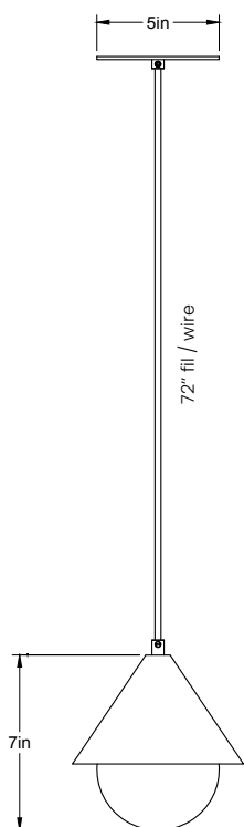
Avant/Front
